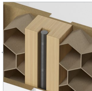
Стабілізатор полотна
